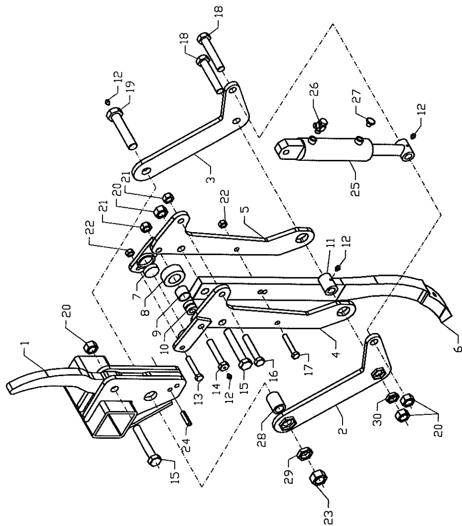
Steinsicherung hydraulisch Komet starr
