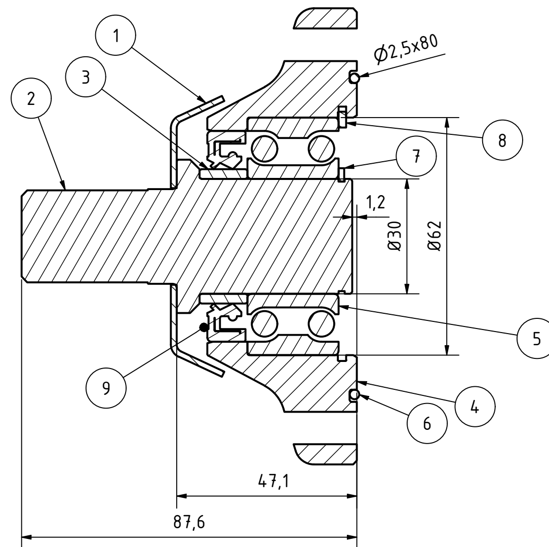
A-A ( 1 : 1 )
