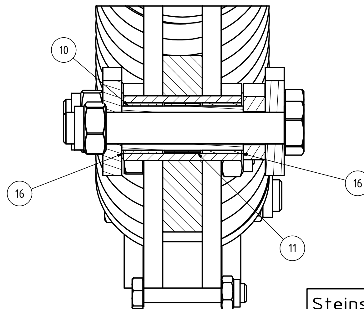
C-C ( 1 : 1,5 )
