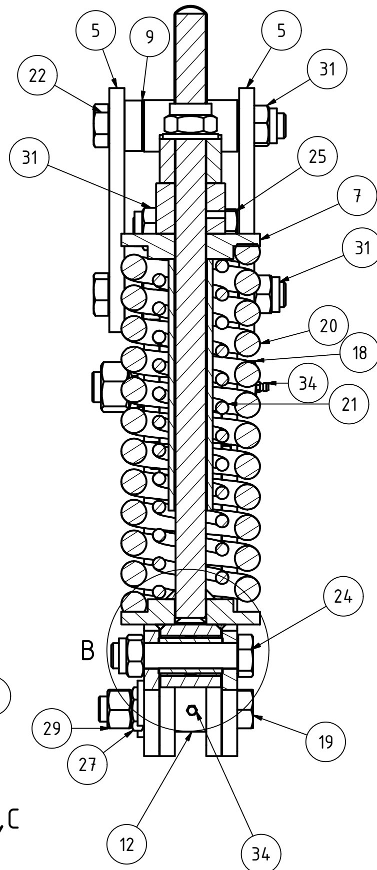
A-A ( 1 : 3 )
